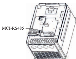
Способ установки MCI-RS485
